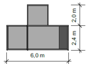
Seitenansicht
